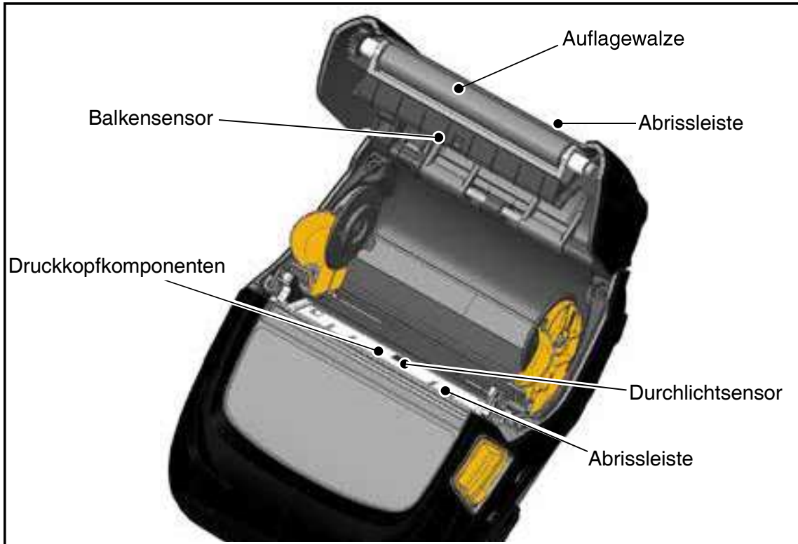
Abbildung 20a: Reinigung der ZQ500 Series-Drucker (Medien mit Trägermaterial)
