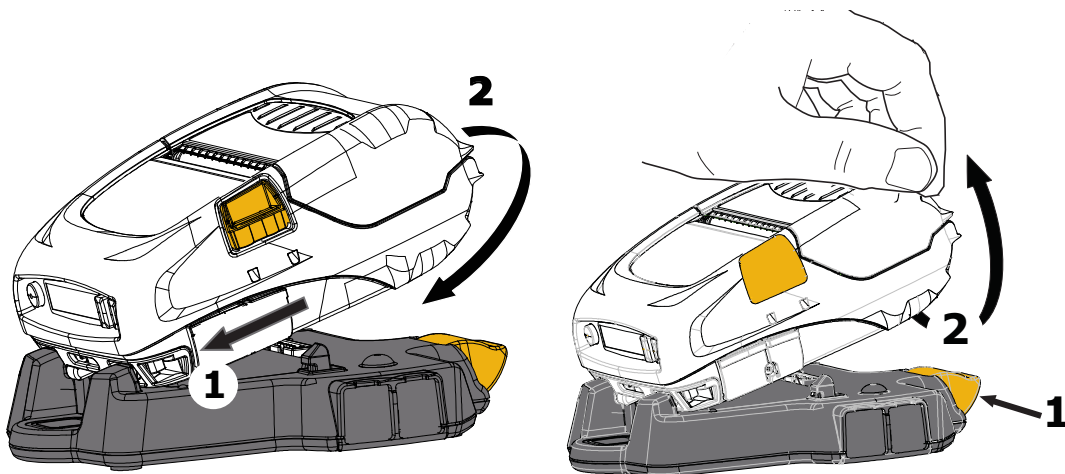
Abbildung 5: Verbinden und Trennen der Fahrzeug-Ladestation
