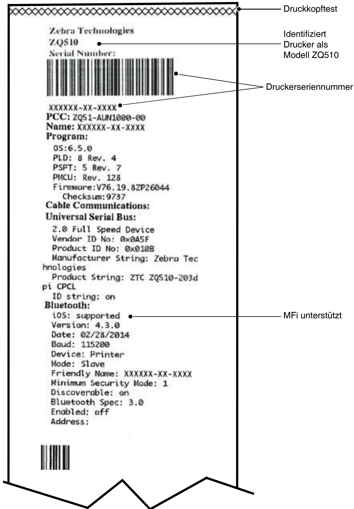
Abbildung 21a: Konfigurationsetikett ZQ500 Series (abgebildet: ZQ510)
