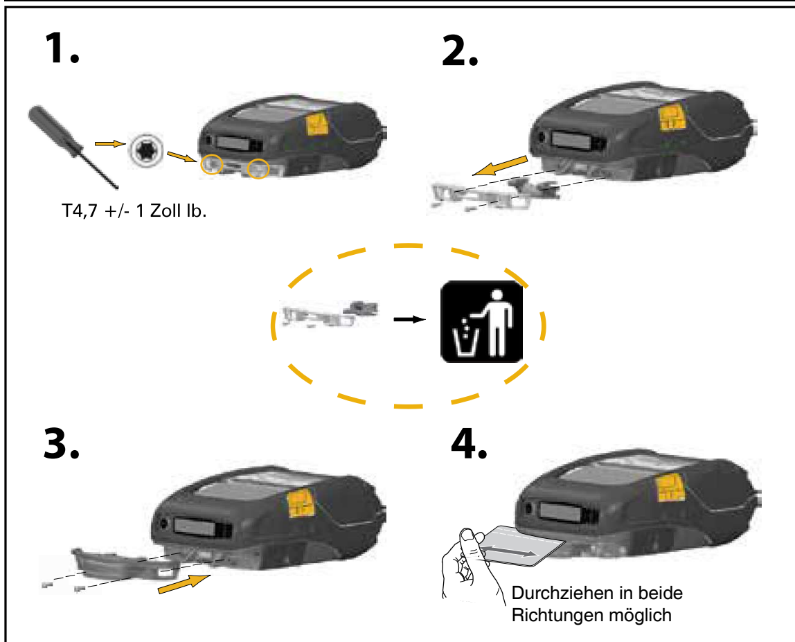
Abbildung 19: Installieren des Magnetkartenlesers
